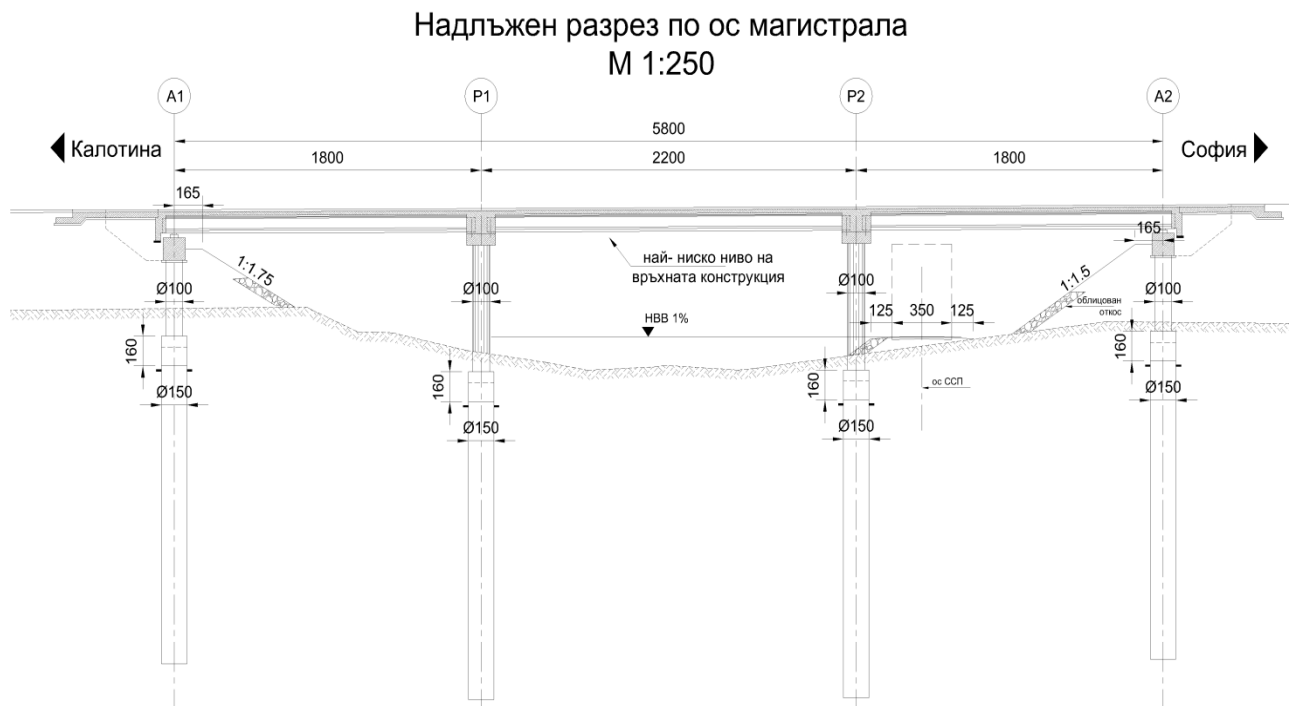
Фигура 4: Надлъжен разрез на моста над р. Белица(р. Костинбродска) при км 38+320 от АМ „Европа“
