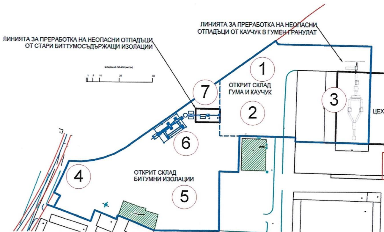
Фигура 2-1 Генплан на новите производствени линии
